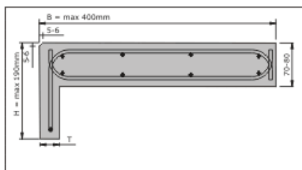
Typ LS mit senkrechter Setzstufe
