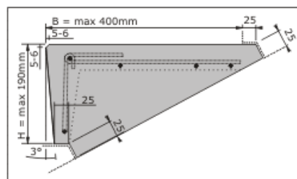
Typ KSS mit hinterzogener Setzstufe
