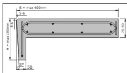
Typ LSS mit hinterzogener Setzstufe
