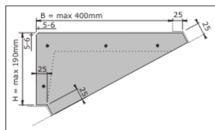
Typ KS mit senkrechter Setzstufe
