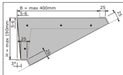
Typ KSS mit hinterzogener Setzstufe
