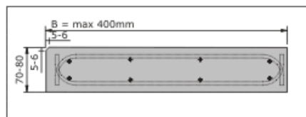
selbsttragende Trittstufe
