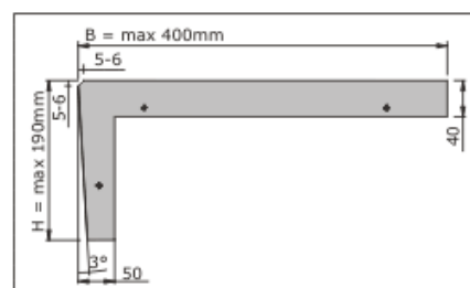
Typ LSS mit hinterzogener Winkelstufe
