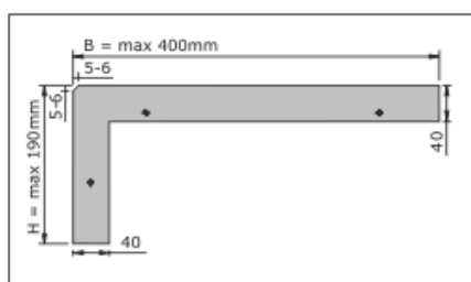
Typ LS mit senkrechter Winkelstufe
