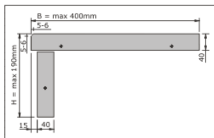
Plattenstufen Typ SD Trittfläche+ Setzstufe
